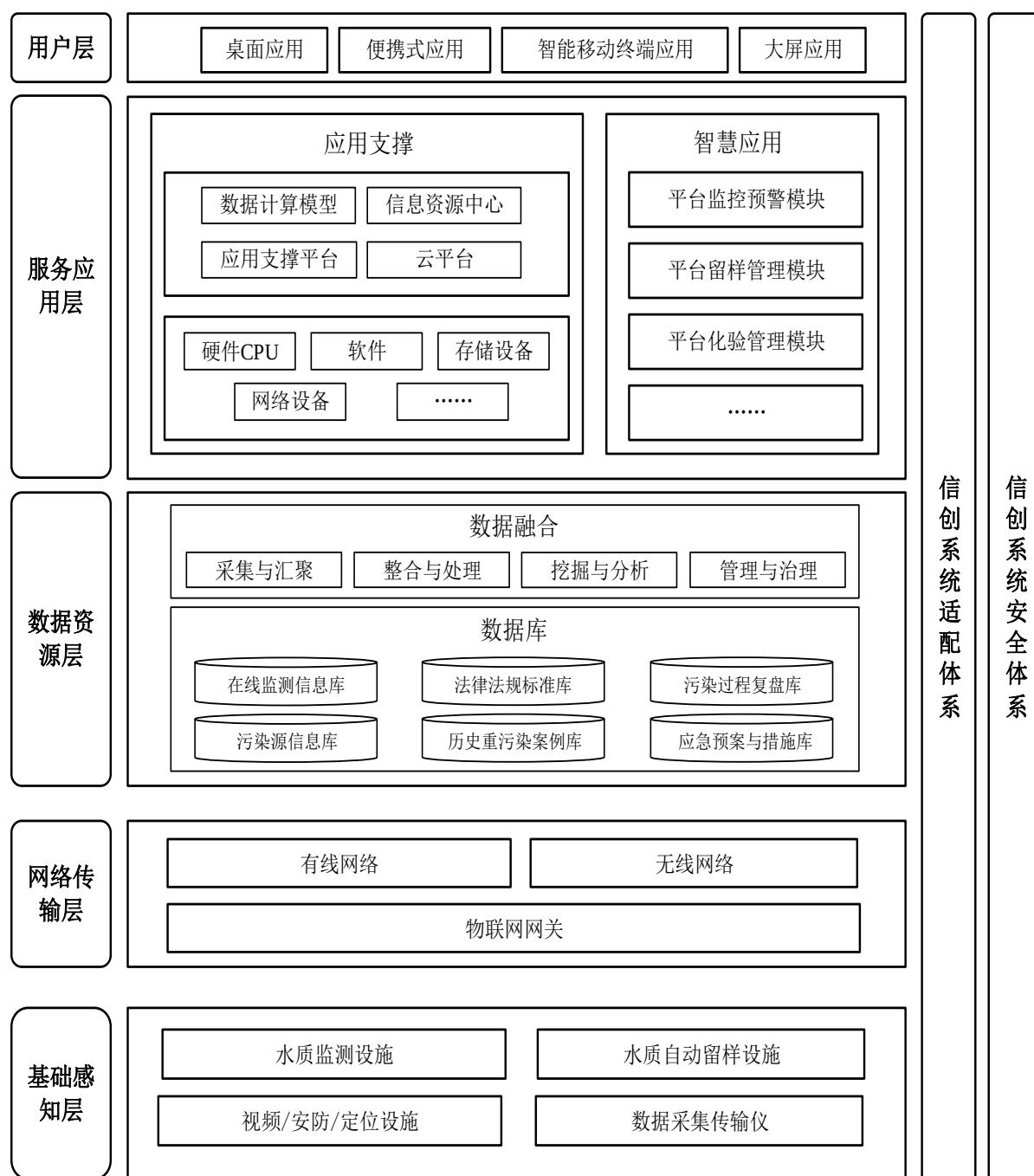
图1 水污染源在线监控系统架构图
